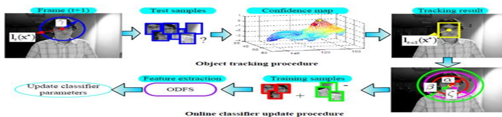
Fig. ODFS tracker
